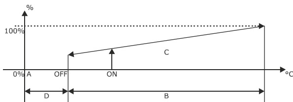
Regolazione con 1 compressore
