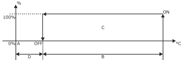
Regolazione con 1 compressore
