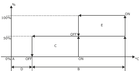
Regolazione con 2 compressori
