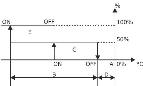
Regolazione con 2 stadi (a 2 gradini)
