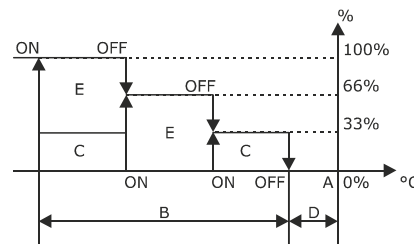
Regolazione con 2 stadi (a 3 gradini)
