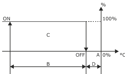
Regolazione con 1 stadio
